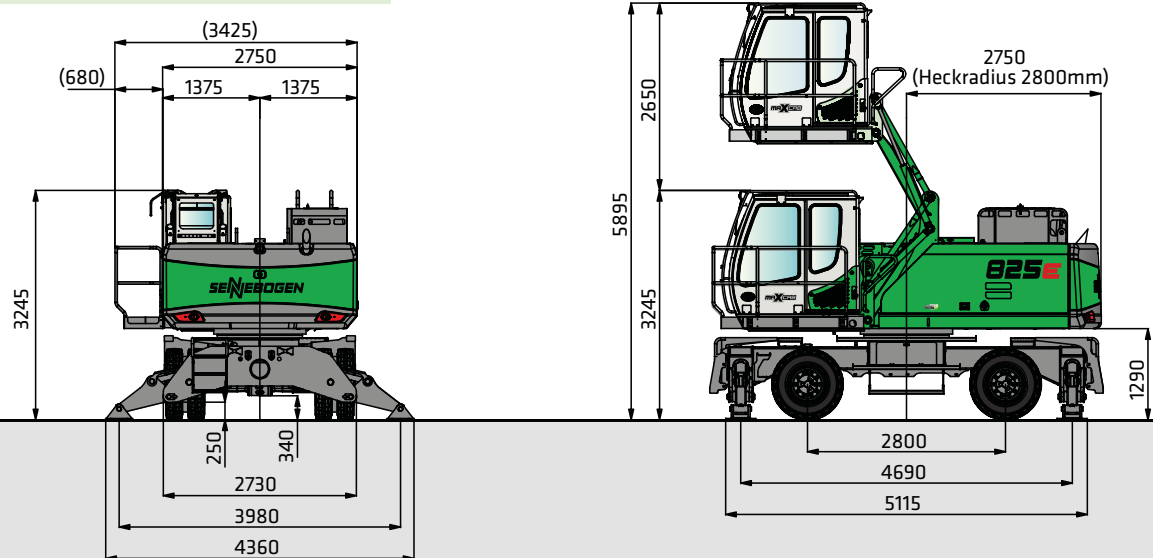
825 M mit Unterwagen Typ MP26 (Serie) und hydraulisch hochfahrbarer Kabine Typ E270
